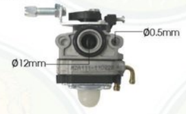
■ HG-139F-08 Carburetor คาร์บูเรเตอร์
