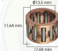
HG52-102 Lower bearings ตลับลูกปืนล่าง
