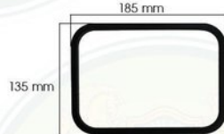
■ KM1100-006 Air filter seal ซีลกรองอากาศ หนา 8 mm
