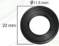
■ HG-CA-018 Sealing ซีลยาง ทน 2.5mm
