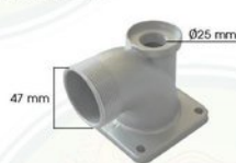
WP15-006 Water outlet 1.5" ข้อต่อน้ำออก 1.5"
