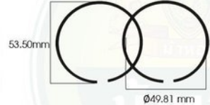
■ HG382-04 Piston ring set ชุดแหวนลูกสูบ
