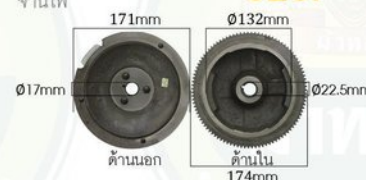
KM2500-47 Fly wheel จานไฟ
