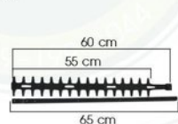
DC600-19 Blade 60cm ใบมีด 60cm
