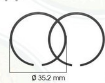
■ HG260-07 Piston ring set ชุดแหวนลูกสูบ
