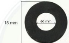
■ HG5.5-40 Gasket ปะเก็น หนา 1mm
