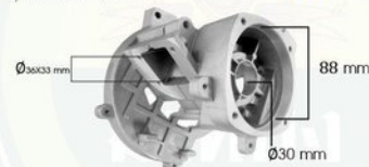
WP20-022 Crankshaft cover ชุดครอบข้อเหวี่ยง
