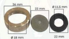
■ HG-CA-004 Spray gun head หัวพ่นยาทองเหลือง
