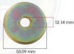
■ HG070-102 Main bearing cover plate ปะกับลูกปืน
