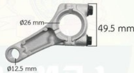
HG64F-03 Connecting rod ก้านสูบ
