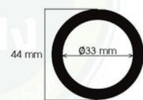
WP15-012 Sealing ซีลกันน้ำ 1.5" หนา 3mm
