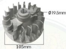
■ HG-139F-06 Fly wheel จานไฟ
