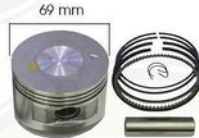
■ HG64F-56 Piston set 1668 ชุดลูกสูบ1668
