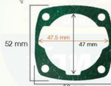
HG767-93 Gasket ปะเก็นเสื้อสูบ
