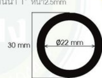
WP10-012 Sealing ซีลกันน้ำ 1" ขนาด 2.5 มม
