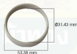
■ HG180-70 Pipe ring แหวนท่อลม
