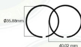
■ HG180-70 Pipe ring แหวนท่อลม
